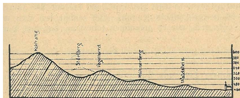
Abb. 19. Schnitt durch das Kohlberggebiet.
